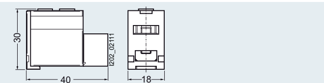
5ST3 770-1HG
