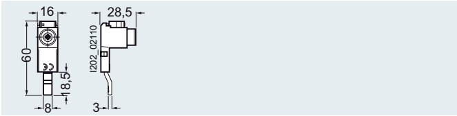
5ST3 770-0HG
