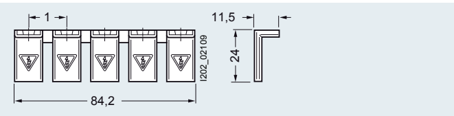
5ST3 655-0HG
