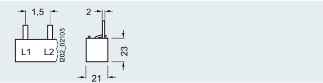
5ST3 710-2HG
