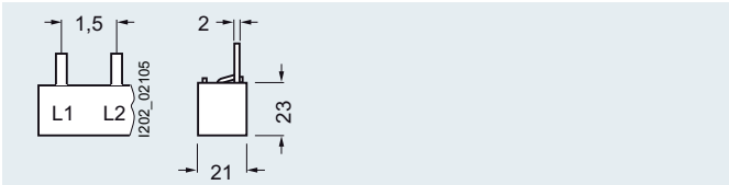
5ST3 705-2HG
